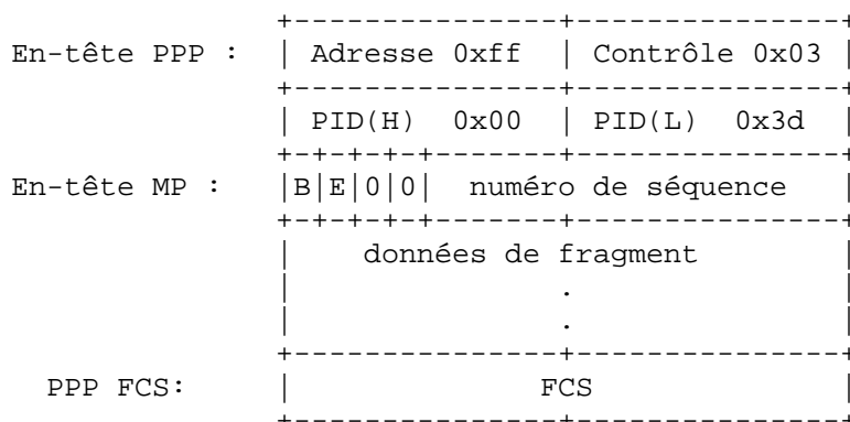
Figure 3 : Format de fragment à numéro de séquence court
