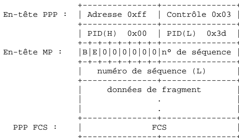
Figure 2 : Format de fragment à numéro de séquence long
