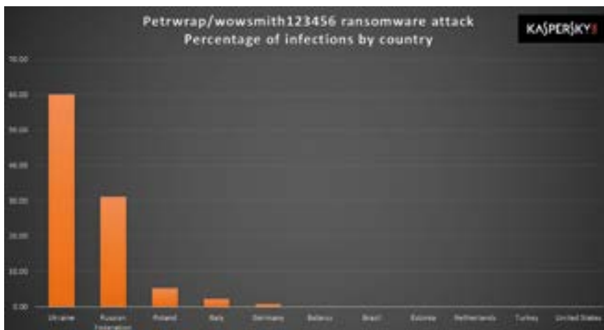
Figure 3 : Pourcentage de machines infectées par NotPetya par pays – Source Kaspersky
